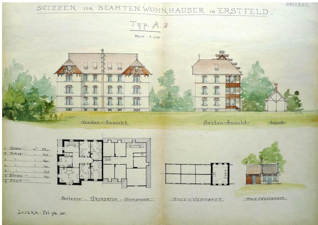
Pläne vom Februar 1894 von Architekten Heinrich Meili-Wapf für Angestellten-Wohnhäuser der Gotthardbahn-Gesellschaft im Mohrenkopf-Quartier in Erstfeld. (Slg. Archiv SBB Historic)
